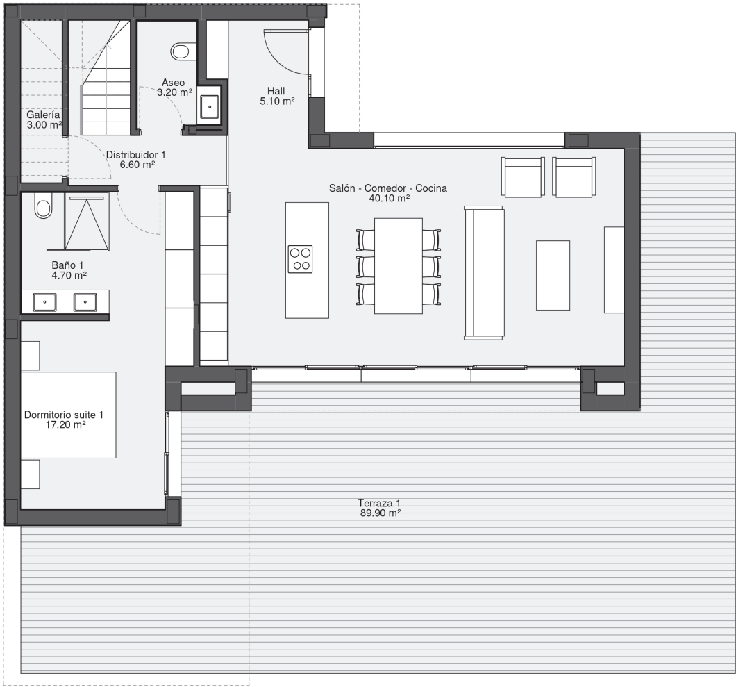
Planta baja
